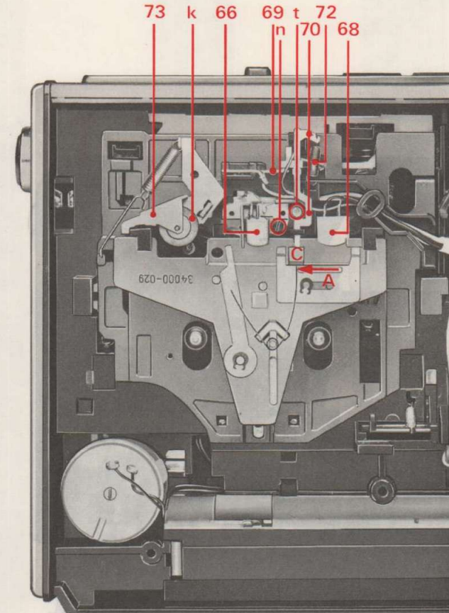
Abb. 5 Kopf justieren Bandendabschaltung einstellen
