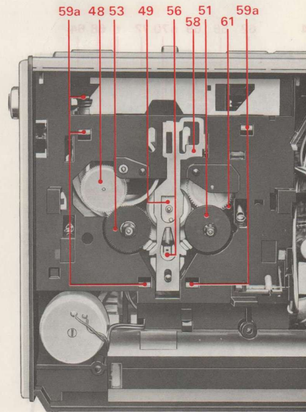
Abb. 8 Schlitten ausbauen
