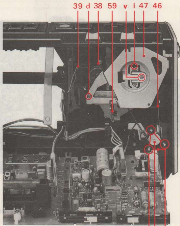
Abb. 6b Tonwelle senkrechtstellen Riemen wechseln Motorbaustein wechseln
