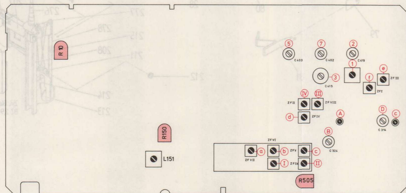
Abgleich-Lageplan ALIGNMENT SCHEME PLAN DE REGLAGE PIANO DI TARATURA
