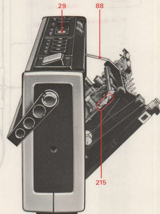
Abb. 3 Vorderwand abnehmen Leiterplatte aushängen Seilzug erneuern
