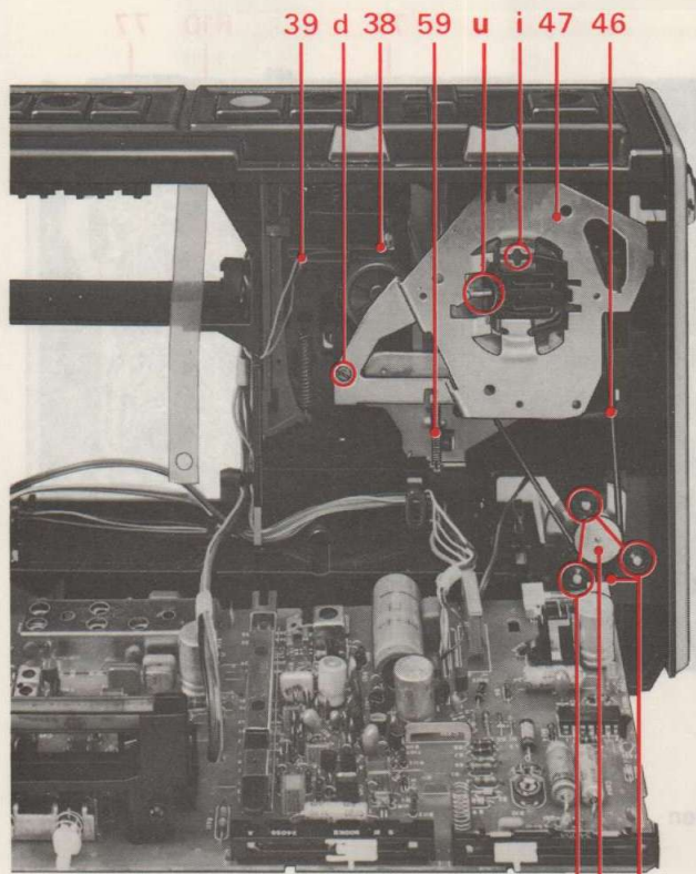
Abb. 6a Tonwelle senkrechtstellen Riemen wechseln Motorbaustein wechseln
